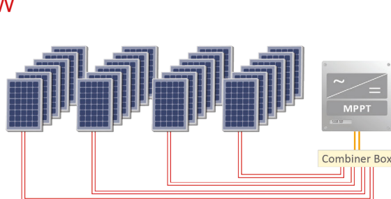
Tradycyjne podłączenie
