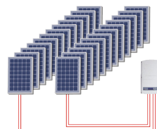
Podłączenie SolarEdge
